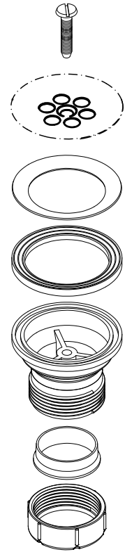
Montaje válvula desagüe Drain valve assembly 1 1/4"
