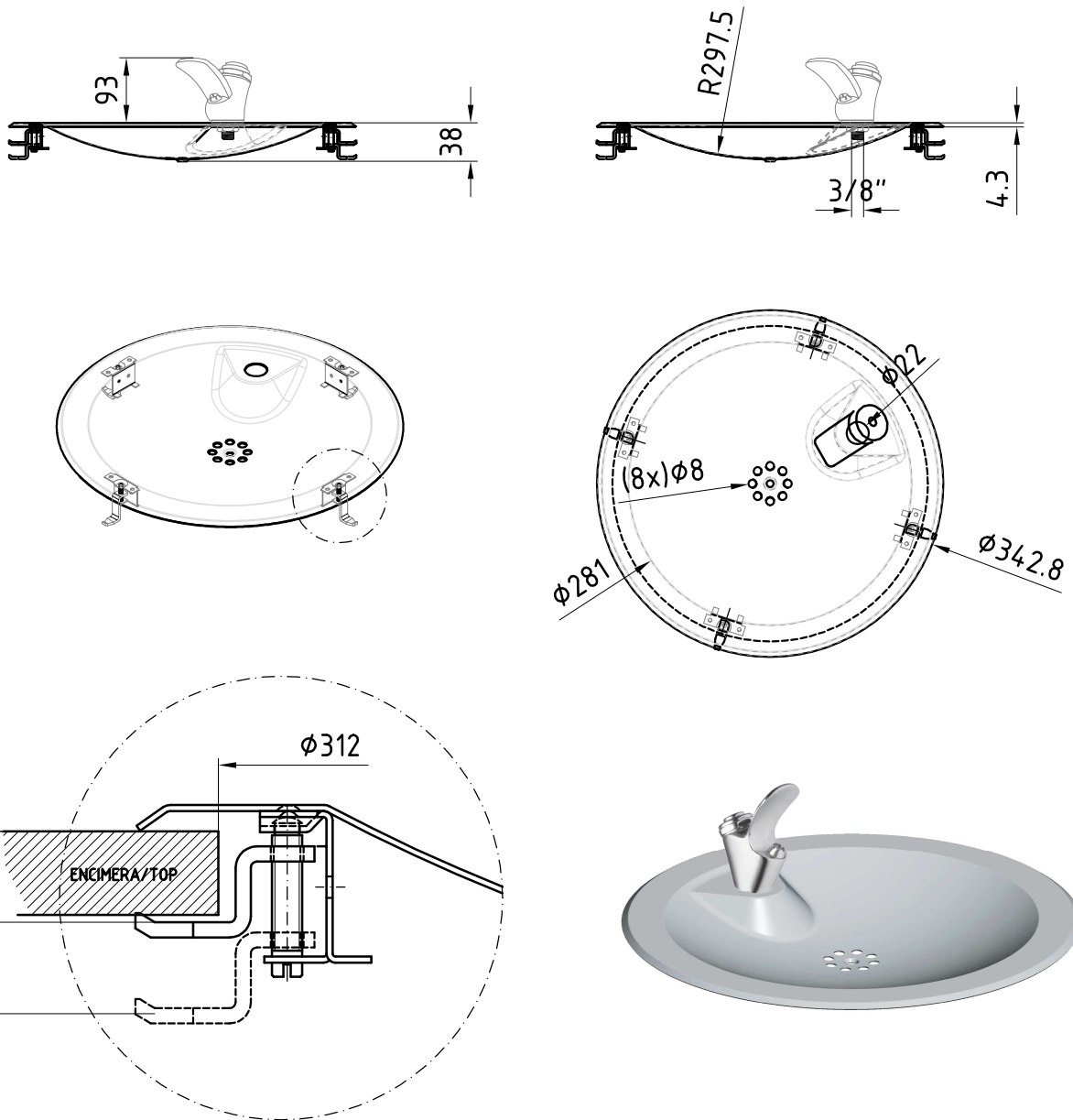
BANDEJA FUENTE AGUA B-FP-E-001
